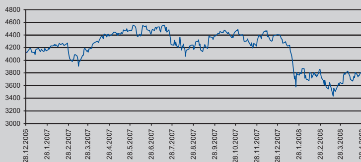
Vývoj hodnoty indexu DJ EuroStoxx50
